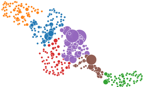
UMAP seed 42
