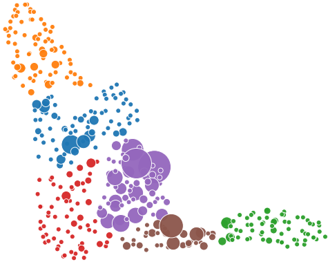
UMAP seed 123
