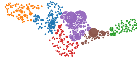
UMAP seed 0
