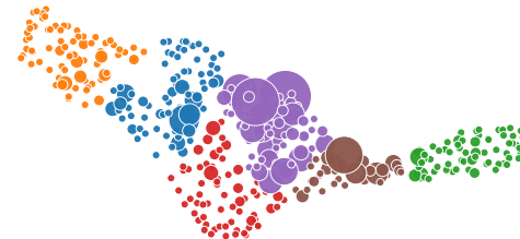
UMAP seed 2024
