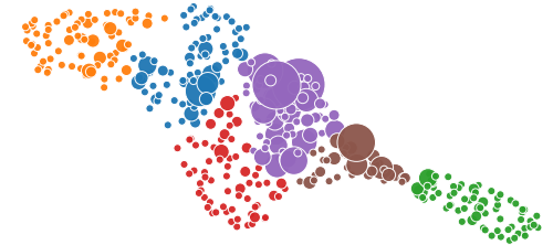
UMAP seed 1
