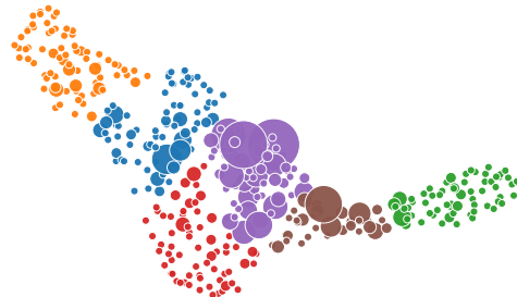
UMAP seed 99
