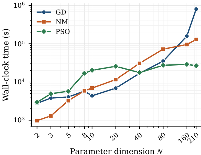
(d) Empirical computational scaling
