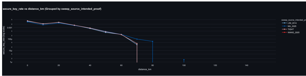
شکل ۲۰.۲۰: مقایسه نرخ کلید امن بر اساس چهار اثبات امنیت مختلف برای پروتکل BB84-Decoy.
