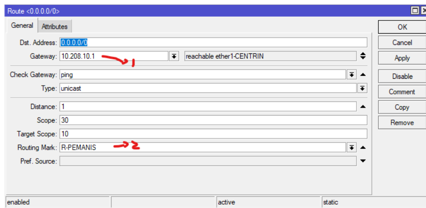
Gambar 7 Konfigurasi Routing Pemanis ke Internet Centrin
