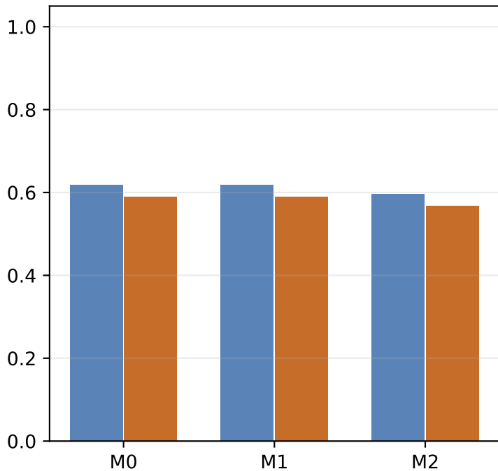
Worst AUPRC
