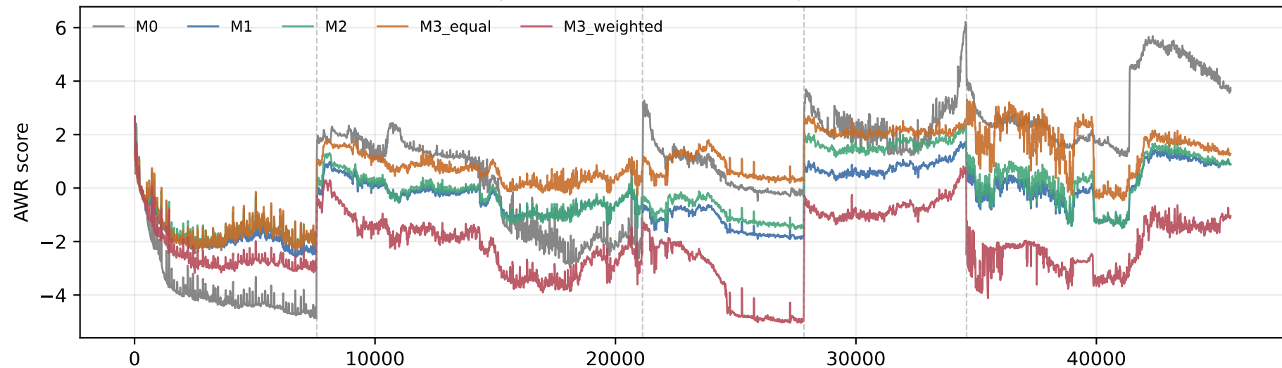
Exp2: M0/M1/M2/M3 AWR trajectories
