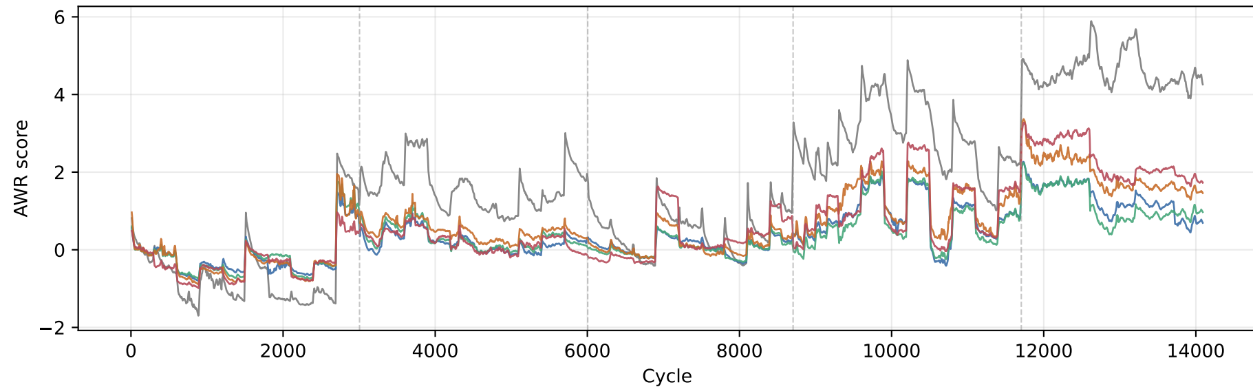
Exp2: M0/M1/M2/M3 AWR trajectories
