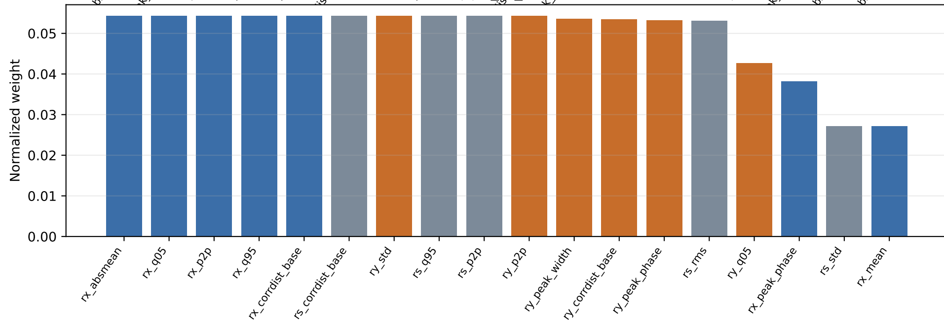
Exp2_to_Exp1
