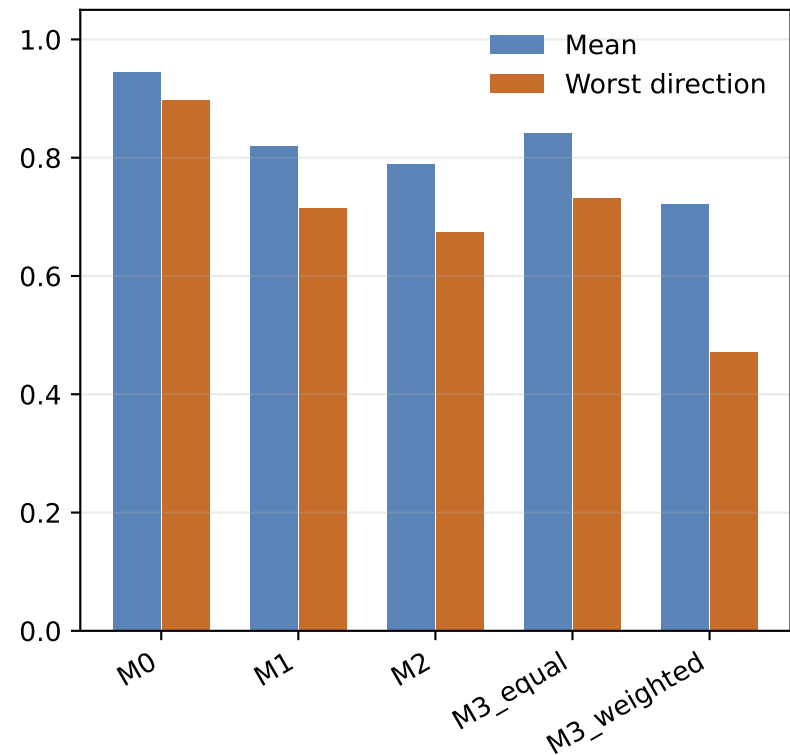
AUROC
