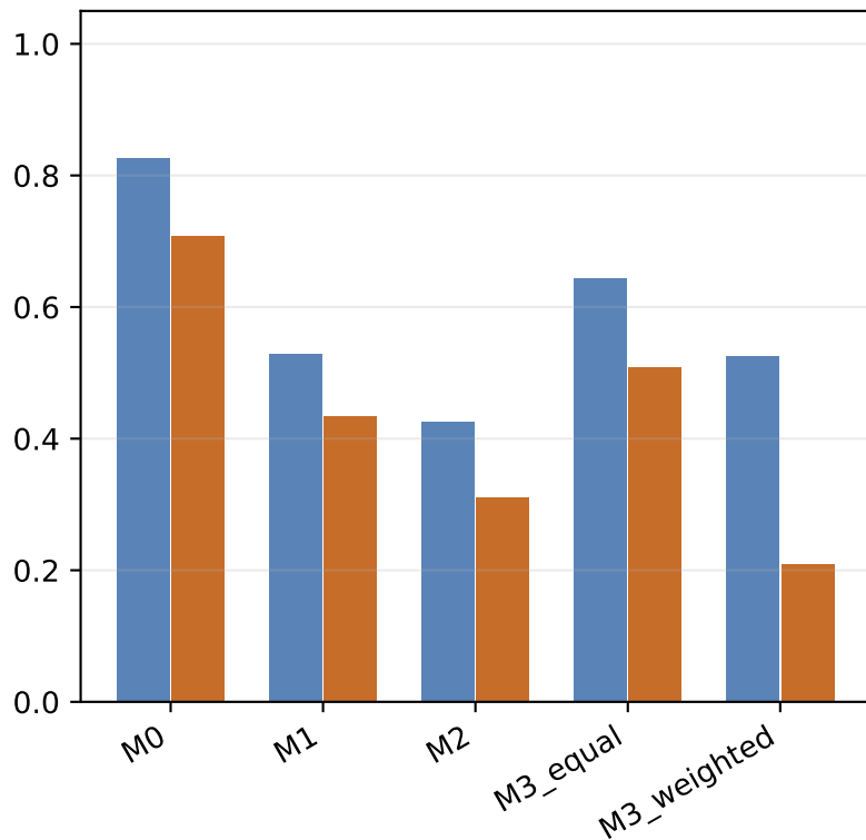
AUPRC
