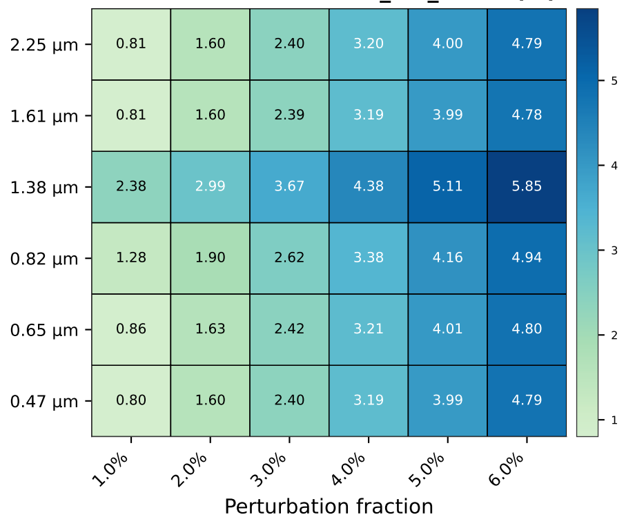
IR B→A — dTb_mean (K)
