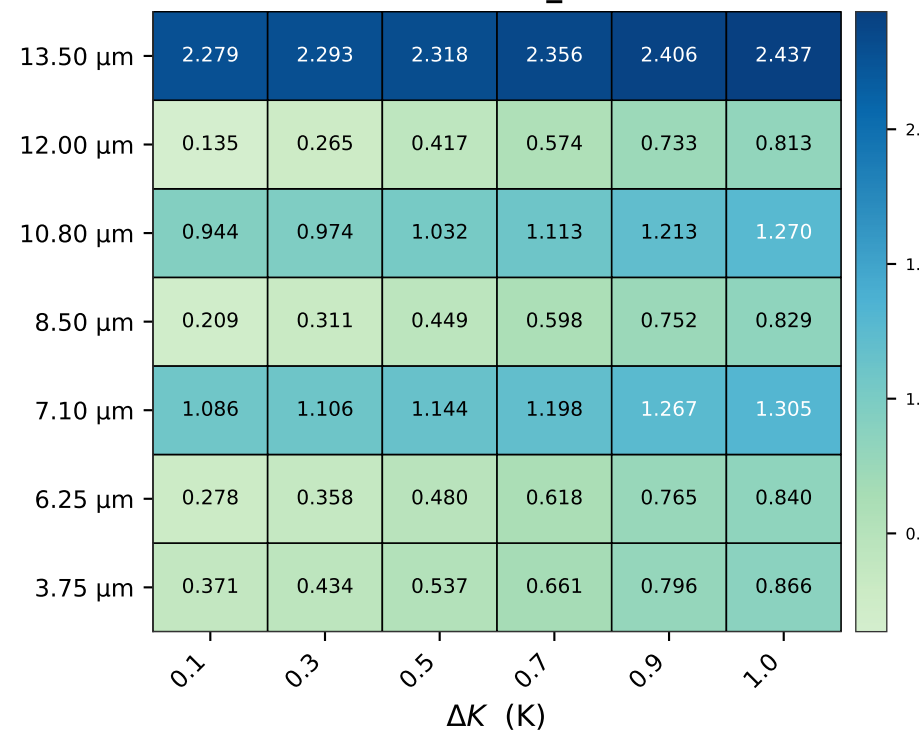
IR A→B — dTb_mean (K)
