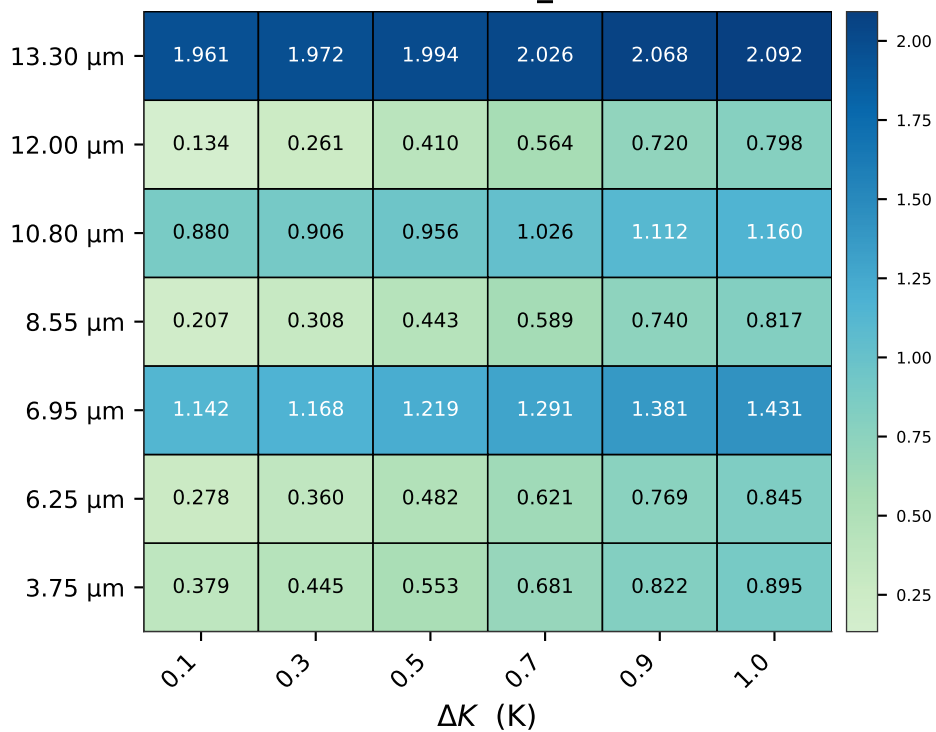
IR B→A — dTb_mean (K)
