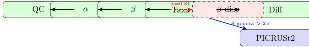
Figure 2: (a) 静的パイプラインは結果に関わらず全ステップを実行。(b) SEQ2PIPE は PERMANOVA 非有意時に \beta フォローアップをスキップし、複数の差次菌属検出時に機能予測を追加する。
