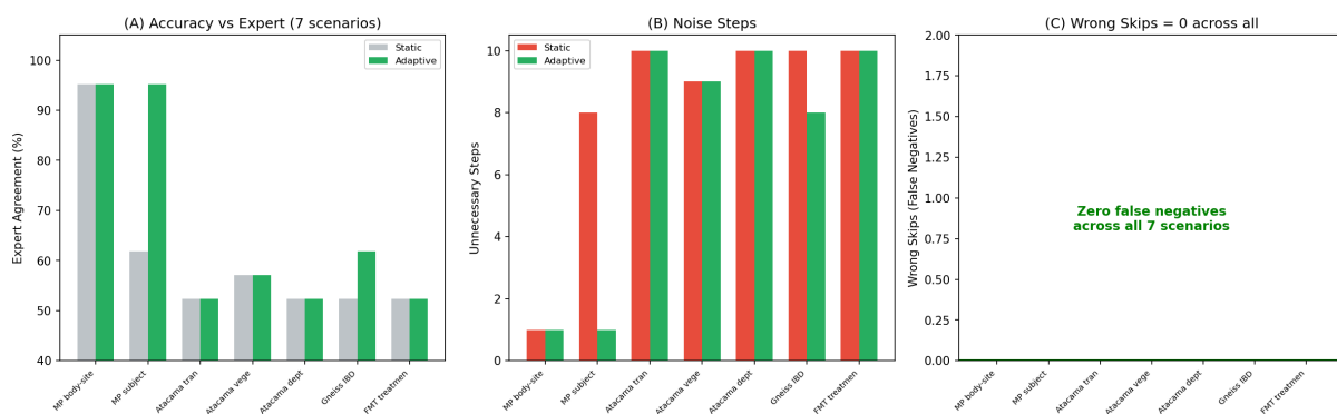
Figure 3: (A) 7 シナリオのエキスパート一致率。(B) ノイズステップ数。(C) 全シナリオで誤スキップ = 0。
