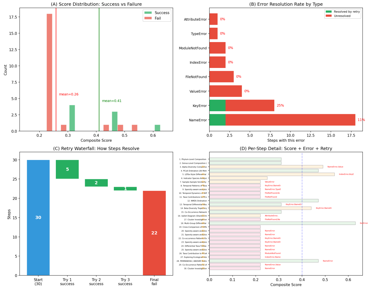
Figure 7: (A) スコア分布。(B) エラー種別解決率。(C) リトライウォーターフォール。(D) ステップ別詳細。
