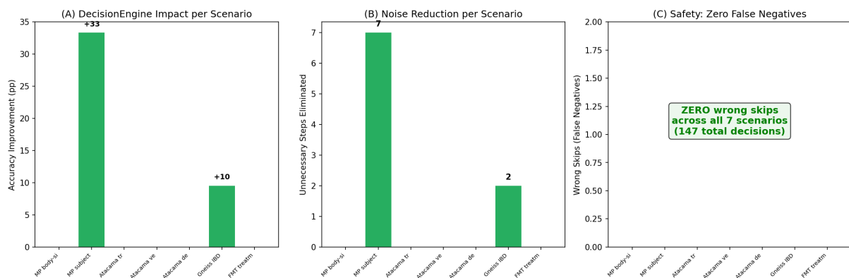
Figure 8: DecisionEngine の影響。(A) 精度改善 (最大 +33pp)。(B) ノイズ除去。(C) 安全性：全 147 判断で誤スキップ =0。
