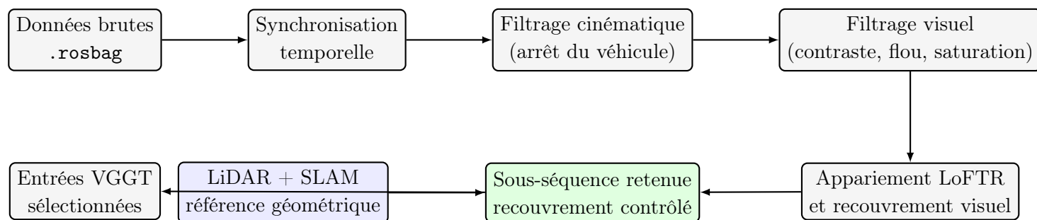
FIGURE 2.3 – Schéma récapitulatif du pipeline de sélection d'images appliqué avant l'alimentation de VGGT.
