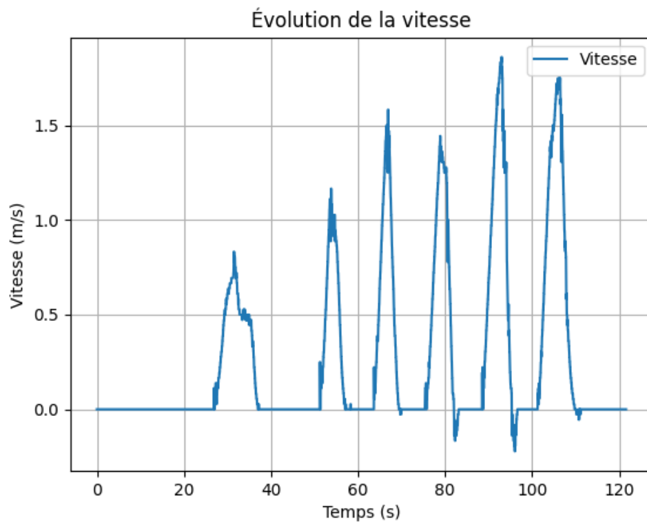
FIGURE 4.5 – Graphique de l'évolution de la vitesse du véhicule, mesurée par les capteurs d'odométrie
