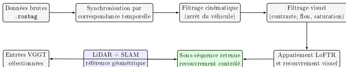
FIGURE 3.1 – Schéma récapitulatif du pipeline de sélection d'images appliqué avant l'alimentation de VGGT.
