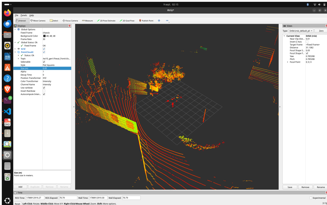
FIGURE 4.4 – Exemple d'acquisition par un capteur LiDAR
