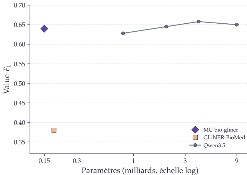
Figure 6: \text{Value-}F_1 sur l'eCRF du lymphome en fonction du nombre de paramètres, après compétition entre les champs.
