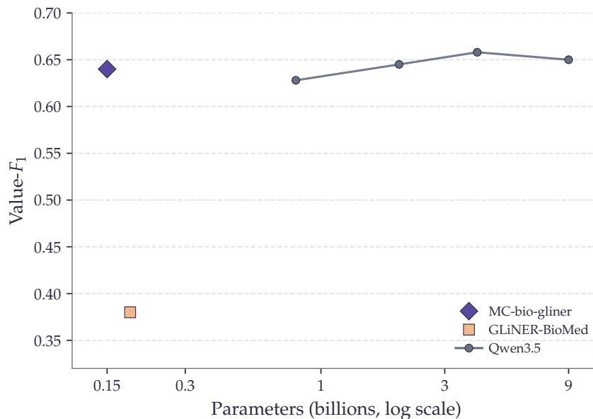
Figure 6: Value- F_1 sur l'eCRF du lymphome en fonction du nombre de paramètres, après compétition des champs. MC-bio-gliner, à 150 millions de paramètres, se situe à 0,018 de valeur- F_1 du meilleur générateur Qwen3.5-4B avec 27 fois moins de paramètres, tandis que la référence GLiNER-BioMed de taille comparable, affinée sur les mêmes dossiers, reste loin derrière.
