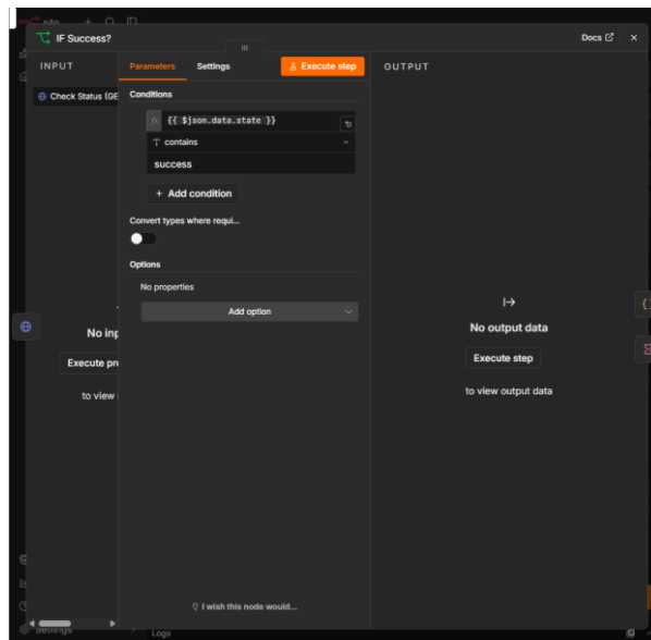
Gambar 6. Kondisi pada node IF Success?
