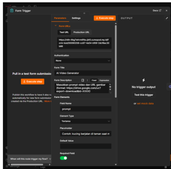
Gambar 2. Konfigurasi node Form Trigger
