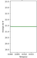
Energie de \psi
