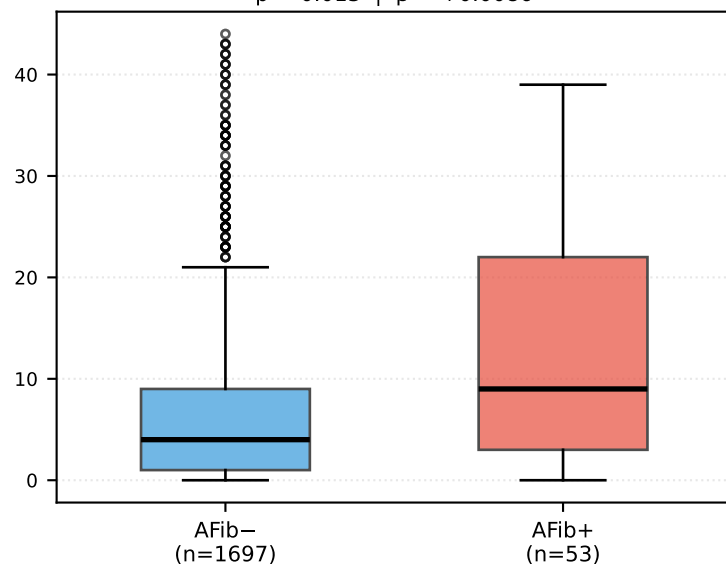
SVES - počet záznamů p = 0.013 | \beta = +0.0086
