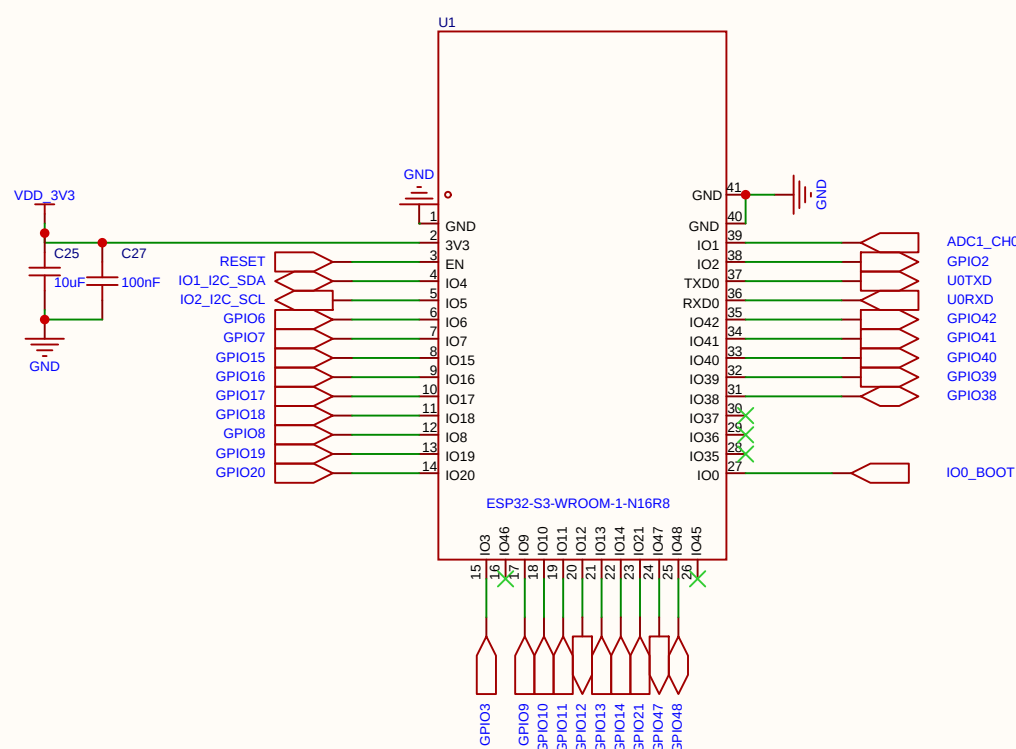
ESP32-S3 8MB PSRAM 16MB FLASH
