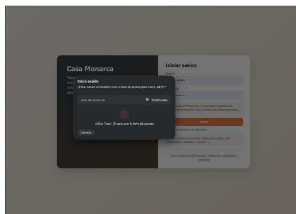
Figura 2: Proceso Passkey
