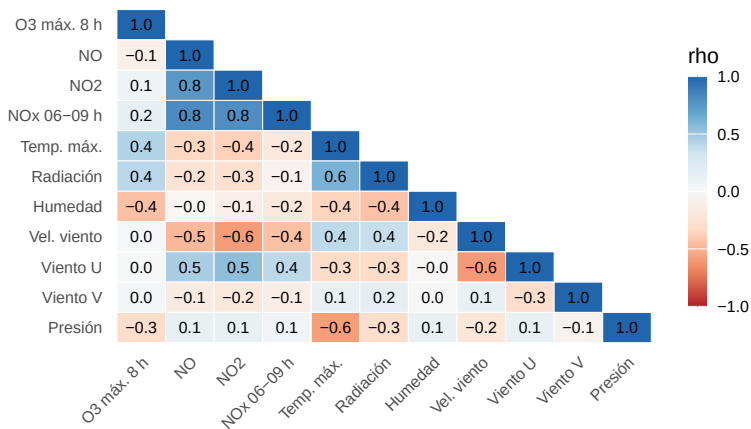
(b) Correlación de Spearman
