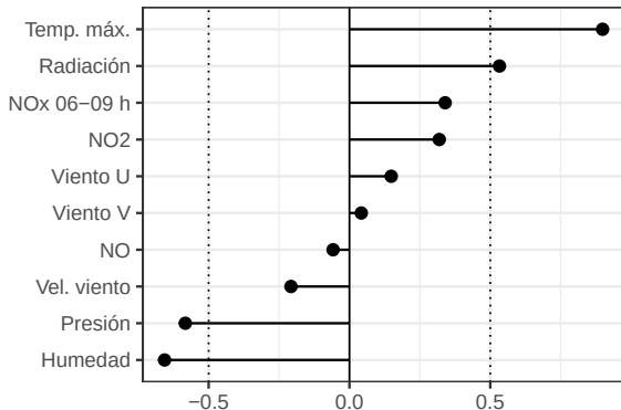
(a) Diferencia entre grupos
