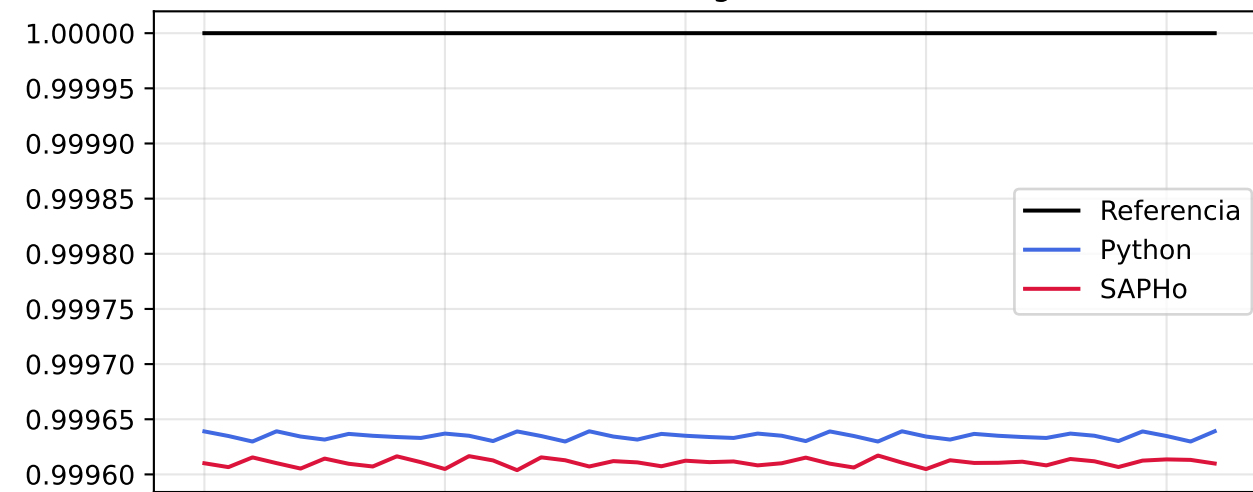
H13 - magnitude
