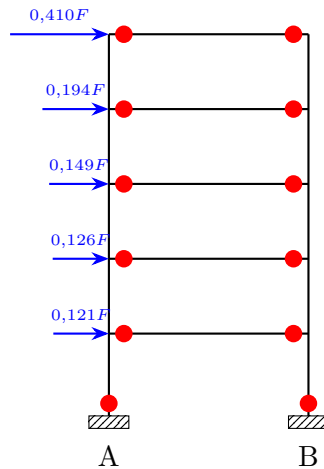
Figura 4: Mecanismo de colapso del eje 2 (rótulas plásticas en rojo).
