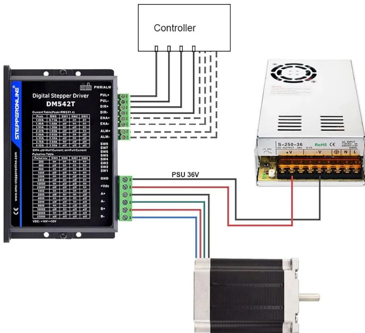
Figura 14 – Diagrama de conexiones para utilizar motor.
