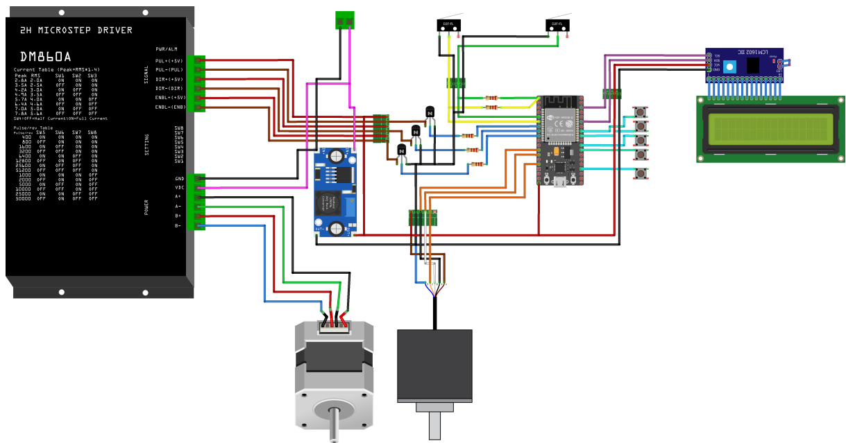
Figura 9 – Diagrama de conexiones de sistema.
