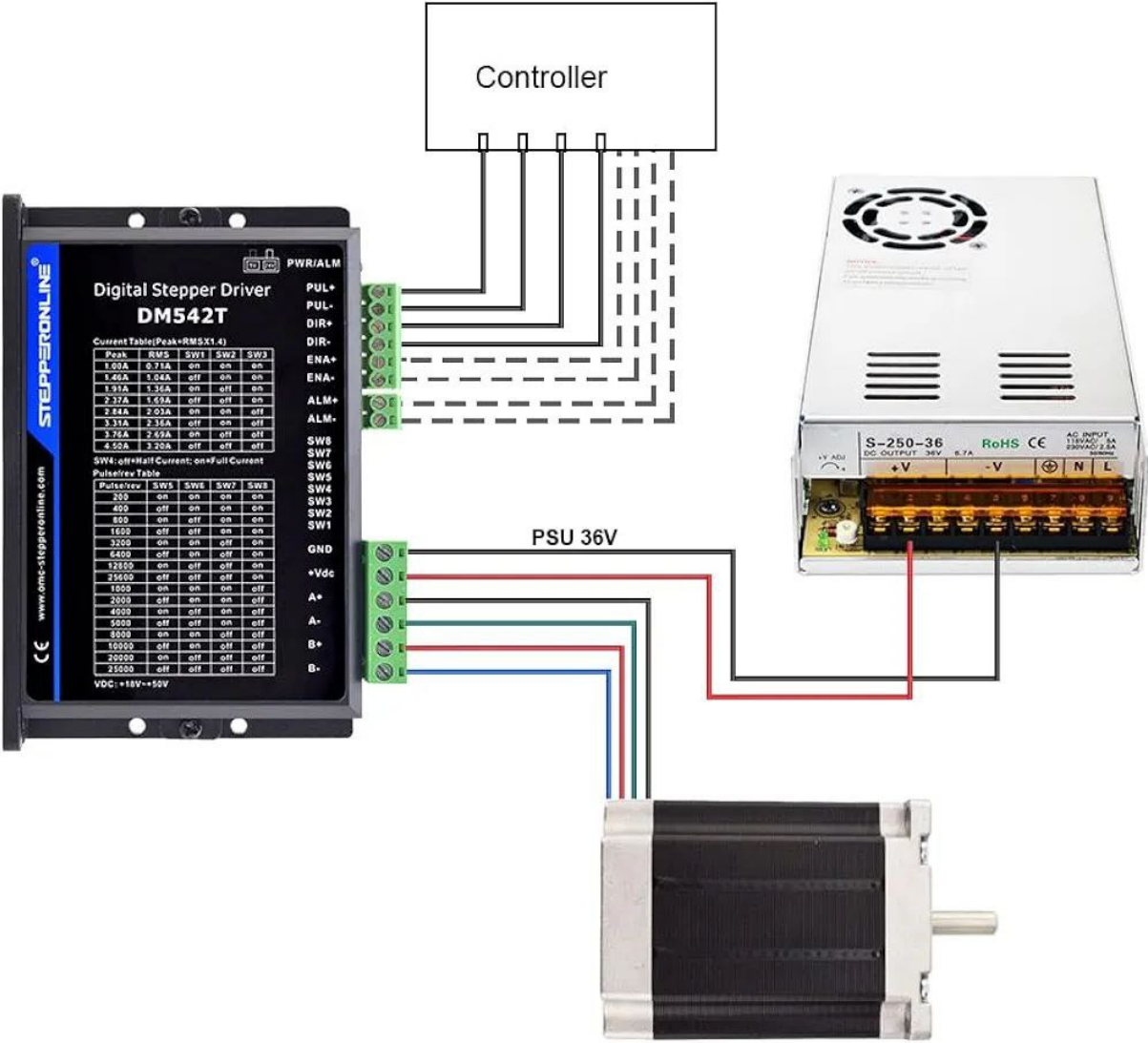
Figura 8 – Diagrama de conexiones para utilizar motor.
