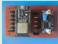
Figura 15: Vista superior de modulo de trabajo basado en esp32.
