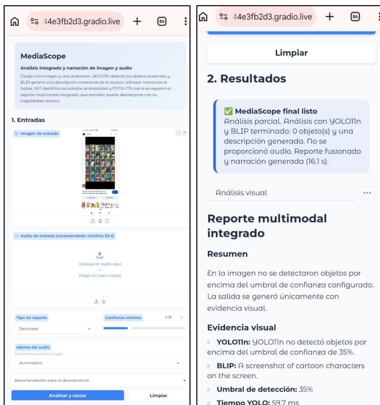
Ilustración 11 Gradio Live
