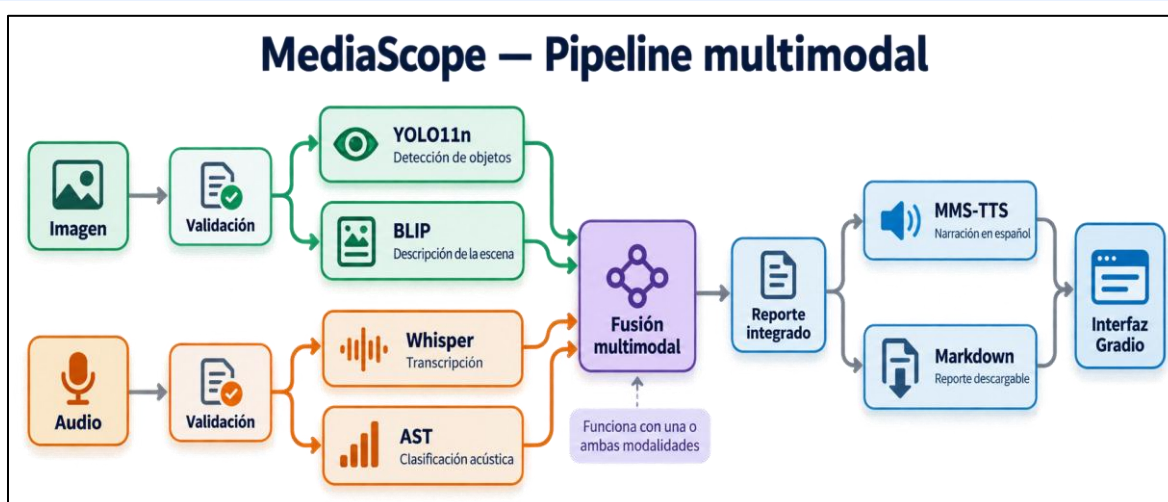
Ilustración 1 Pipeline_General App
