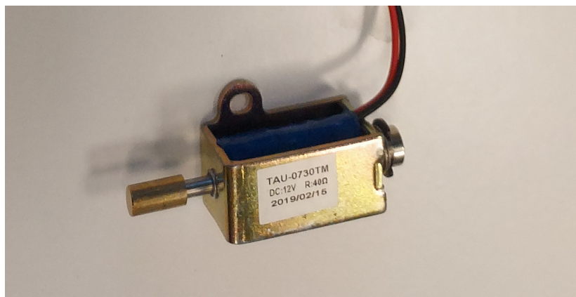
Figura 2: Elettromagnete solenoide TAU-0730TM.
