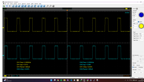
Figura 3: (Stato finale dopo calibrazione: entrambi i canali a f = 2.000 \text{ kHz} , V_{pp} \approx 3.5 \text{ V} , T = 500 \mu\text{s} , duty cycle 24.8%, Scala 500 \mu\text{s/div} .)
