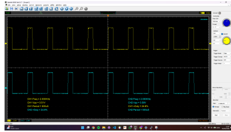
Figura 3: ( Stato finale dopo calibrazione: entrambi i canali a f = 2.000 \text{ kHz} , V_{pp} \approx 3.5 \text{ V} , T = 500 \text{ } \mu\text{s} , duty cycle 24.8\% , Scala 500 \text{ } \mu\text{s/div} .)
