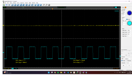
Figura 2: Configurazione iniziale: CH1 con segnale a bassa ampiezza ( V_{pp} = 188 \text{ mV} , \text{RiseT} = 104 \text{ } \mu\text{s} ). Scala 1 \text{ ms/div} , trigger su CH2.
