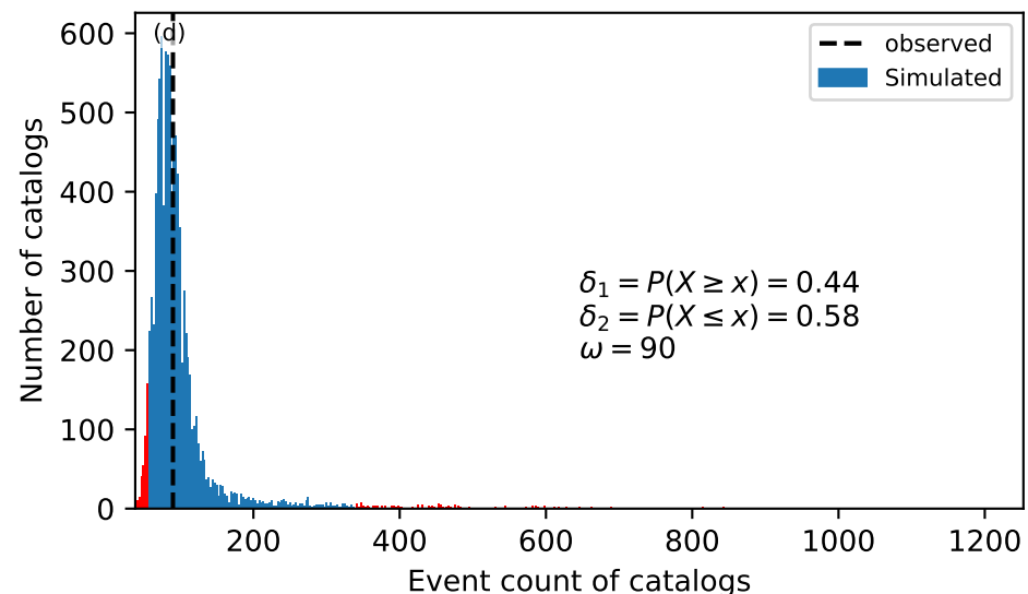
N-Test
