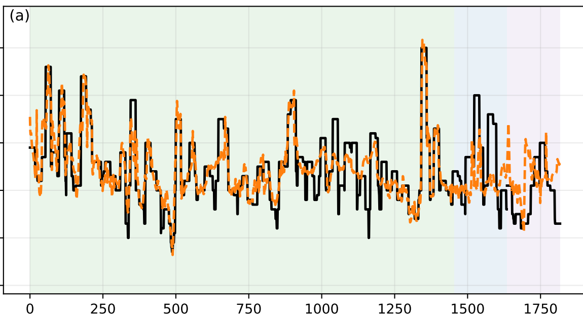
EM-EQF (+log( \Delta t ))
