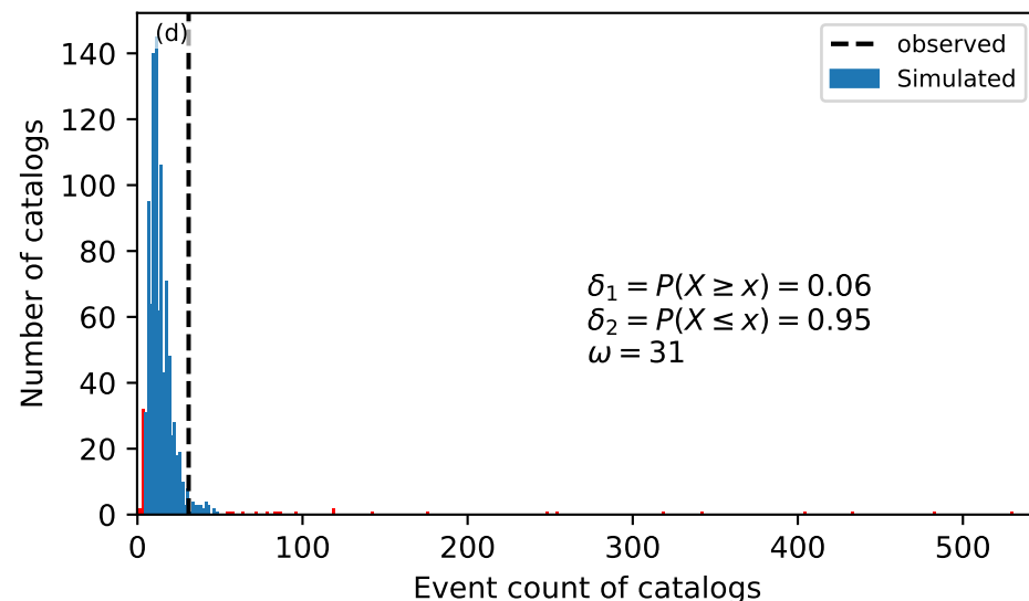
N-Test
