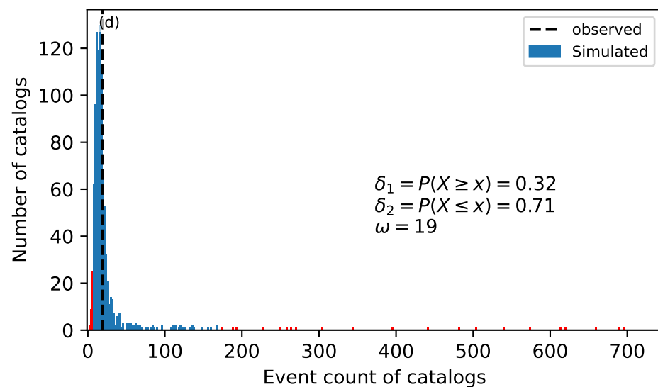
N-Test
