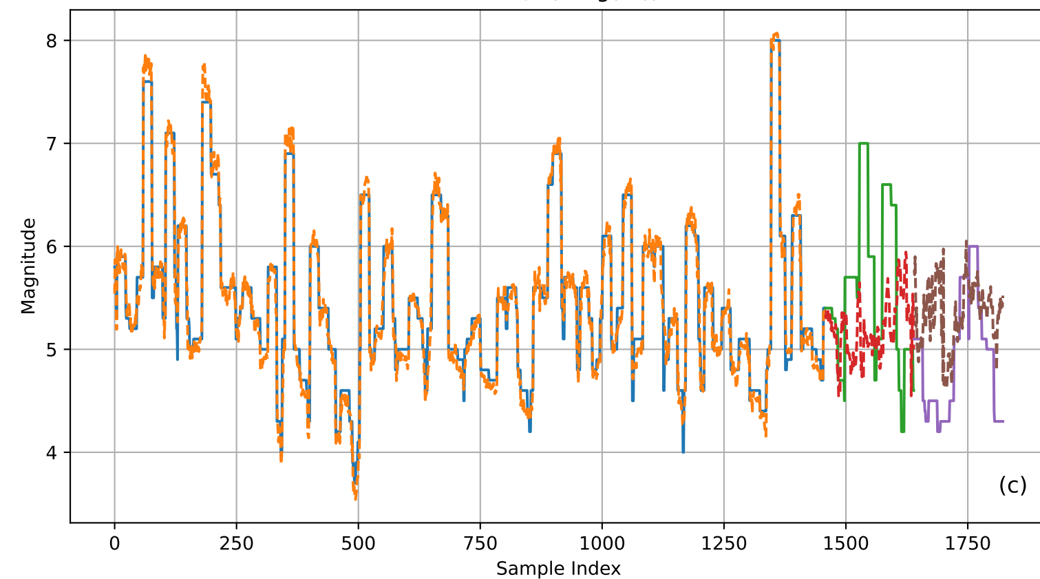
EM-EQF (-TMAP)
