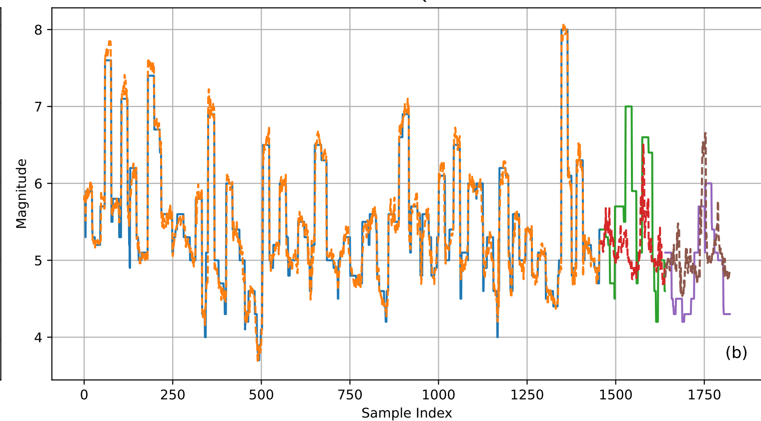
EM-EQF (-T-XPOS)
