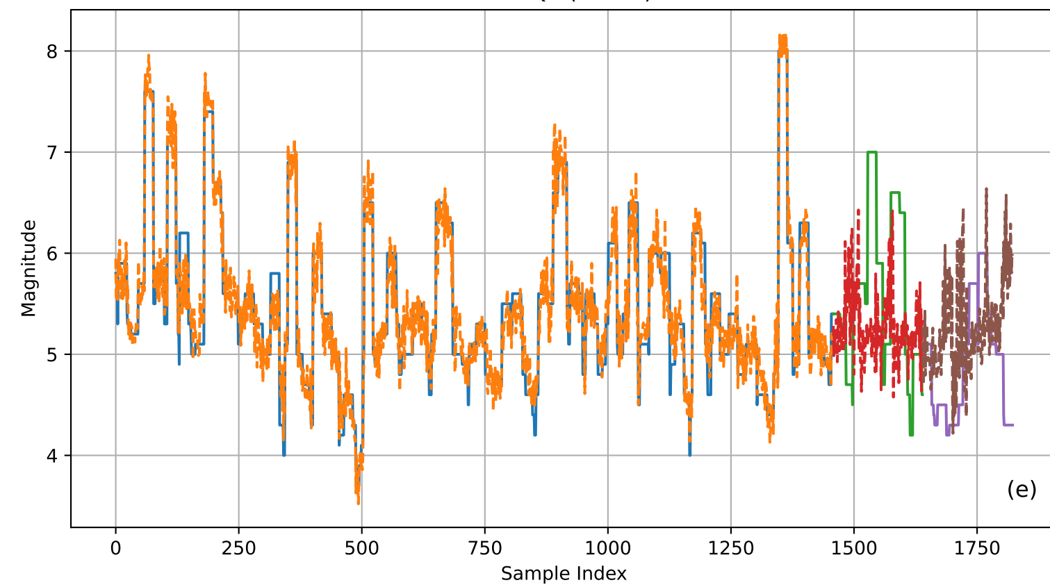
EM-EQF (-TMAP)
