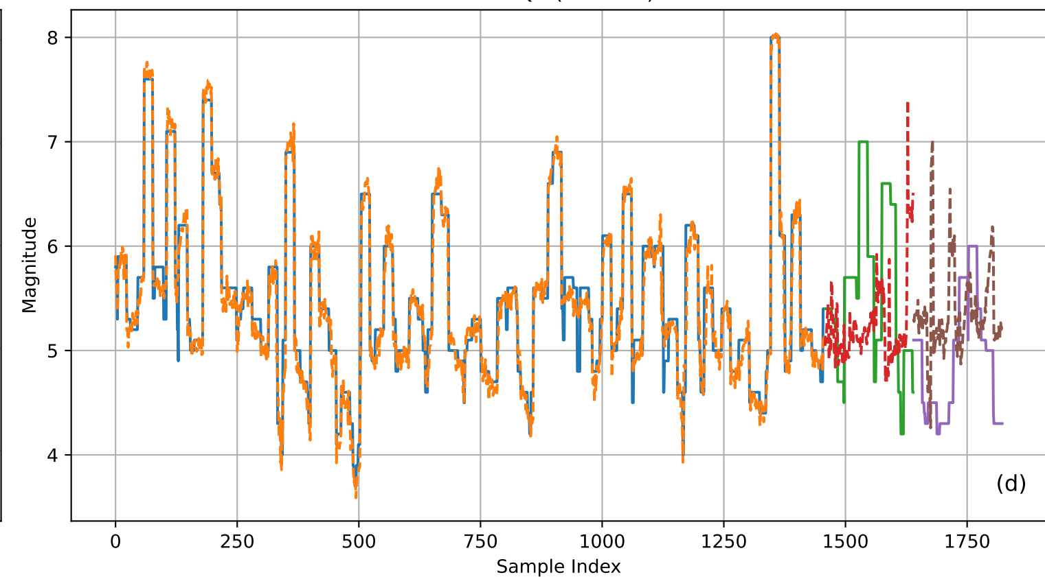
EM-EQF (-Pretrain)
