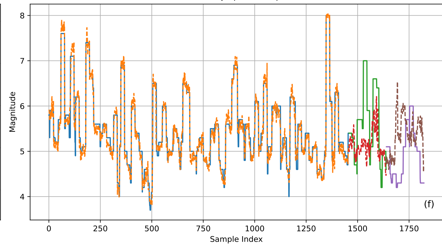
EM-EQF (-Pretrain)
