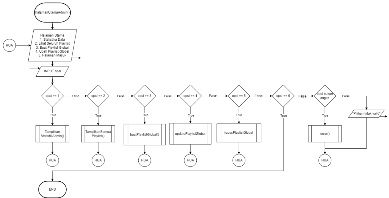
Gambar 2.3 Flowchart Halaman Utama Admin
