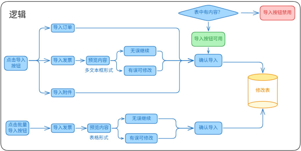
图 7: 导入逻辑草图
