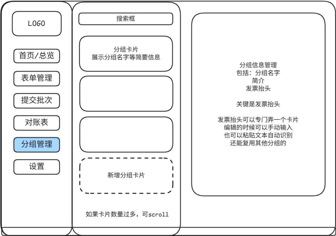
图 12: 分组管理草图
