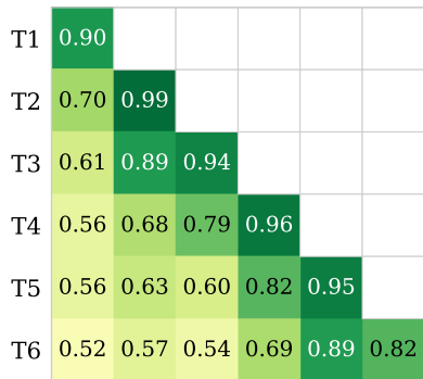
ERO-MoE-CIL
