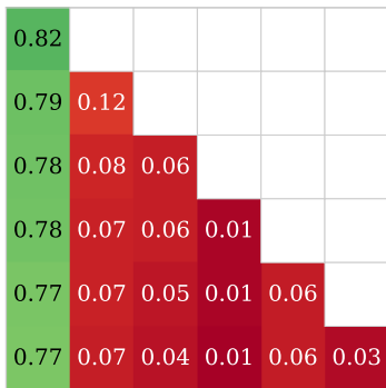
L2P
