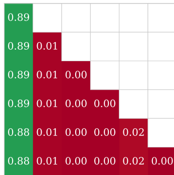
CodaPrompt
