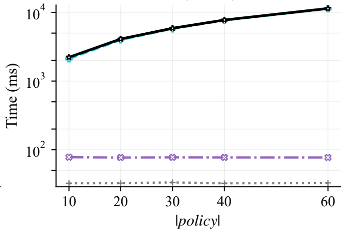
A1 (ss1024)
