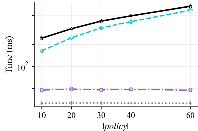
MNT224
