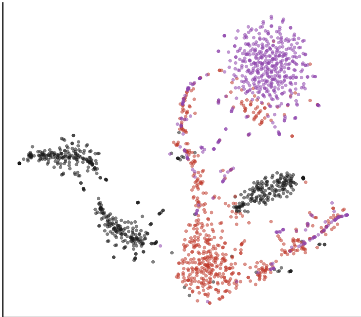
t-SNE
