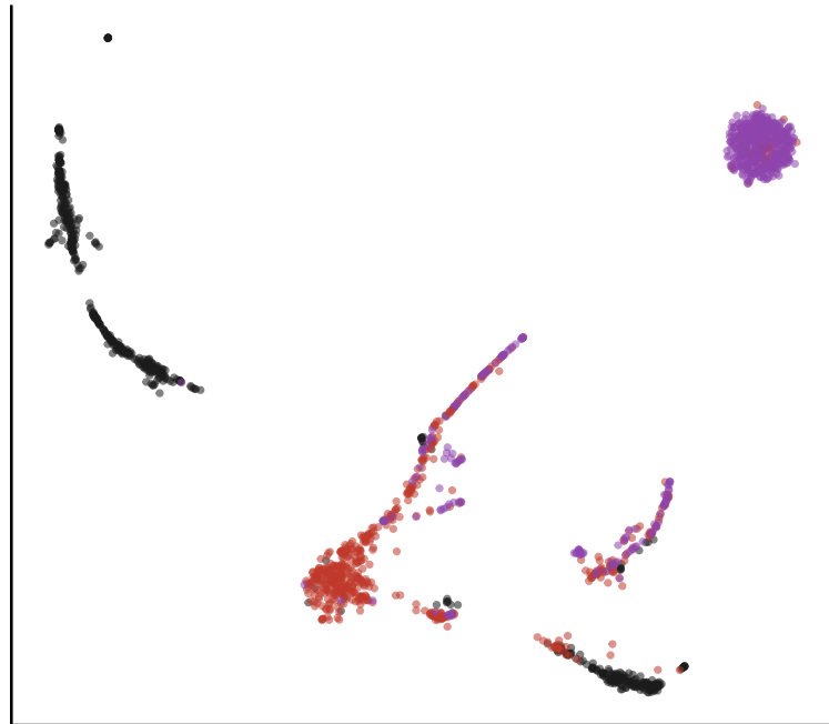
UMAP
