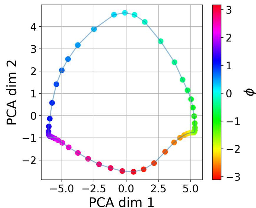
Softsign-shift
