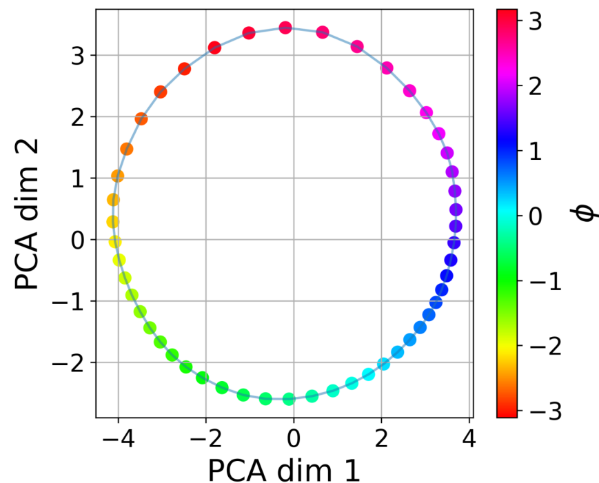
Tanh
