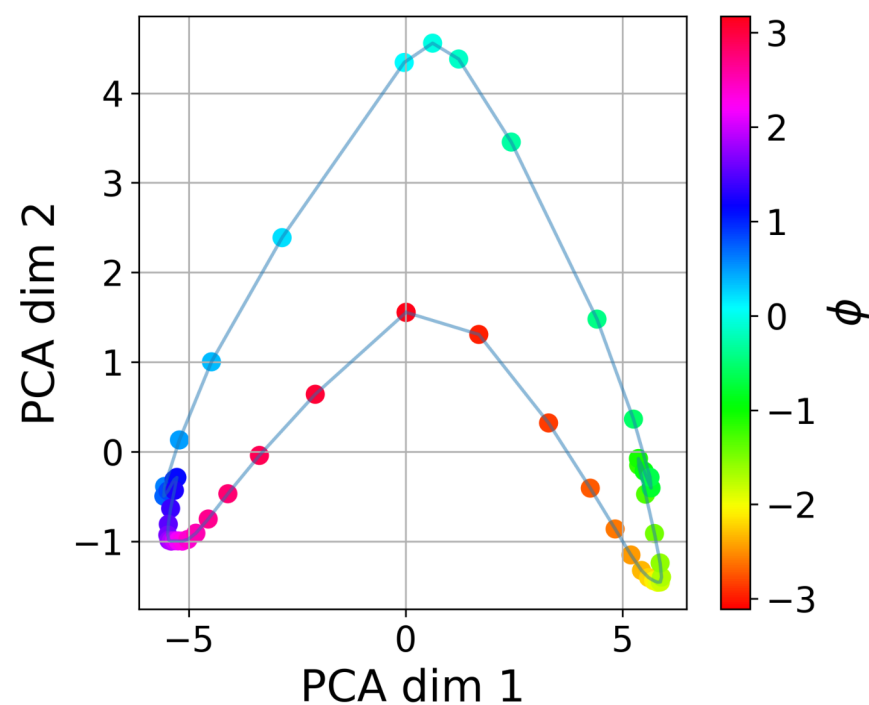
Sigmoid
