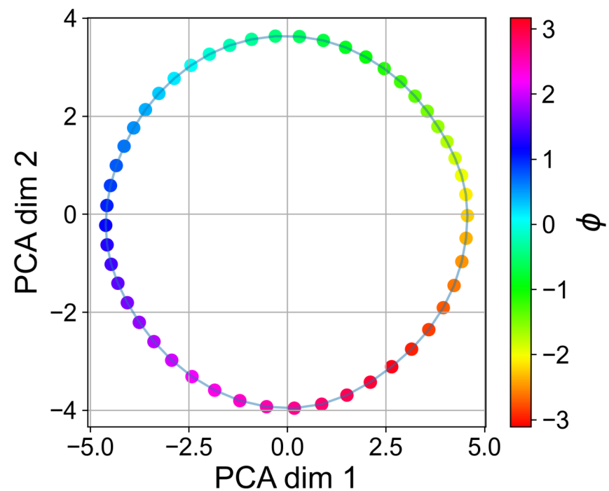
Softsign
