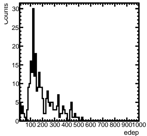
10MeV
