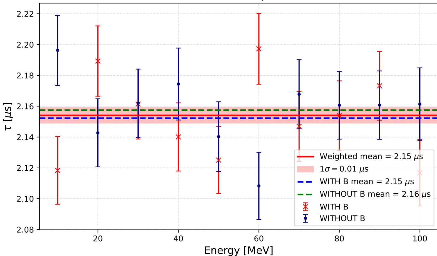
Muons lifetime per run
