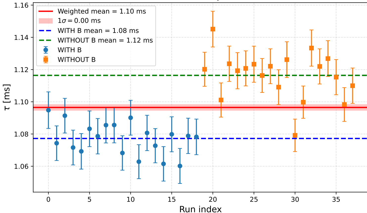
Muon lifetime per run
