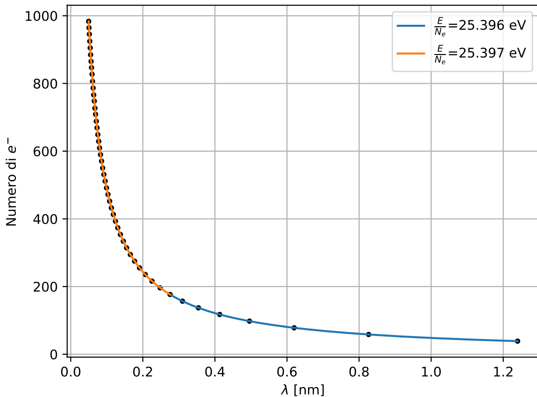
Numero di elettroni vs \lambda
