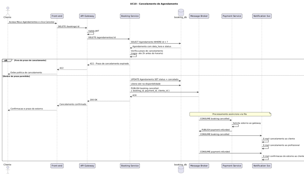
Figura 14 – diagrama de sequência: cancelamento do agendamento
