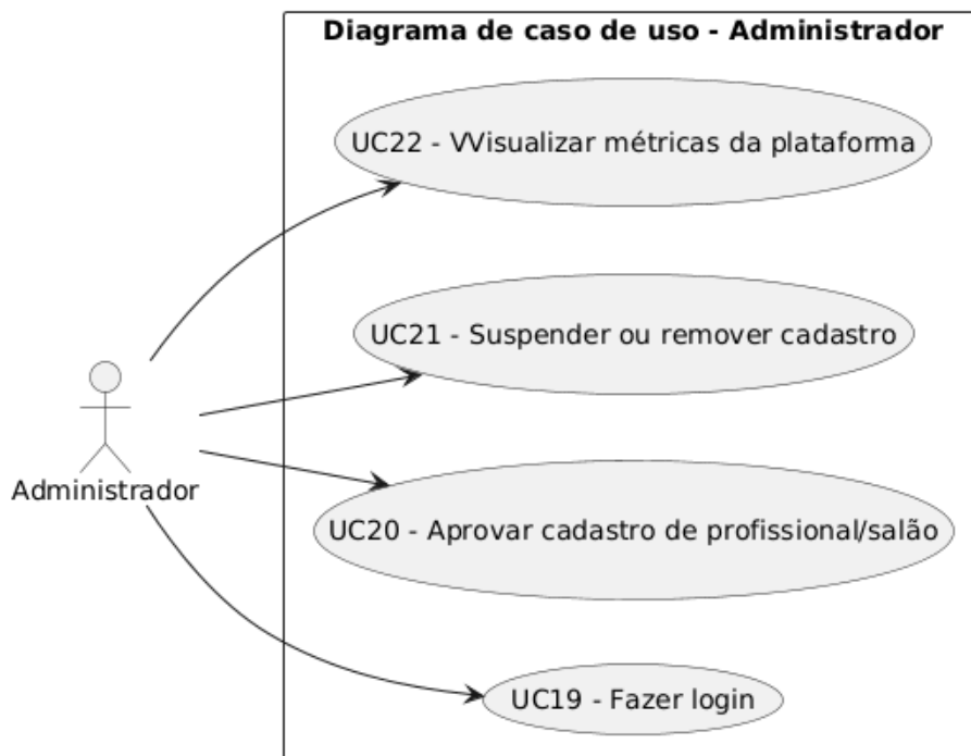
Figura 9 – Diagrama de Casos de Uso: Administrador
