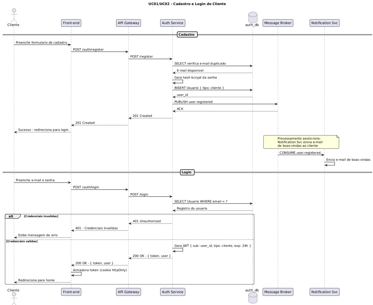
Figura 11 – diagrama de sequência: fluxo de cadastro e login do cliente
