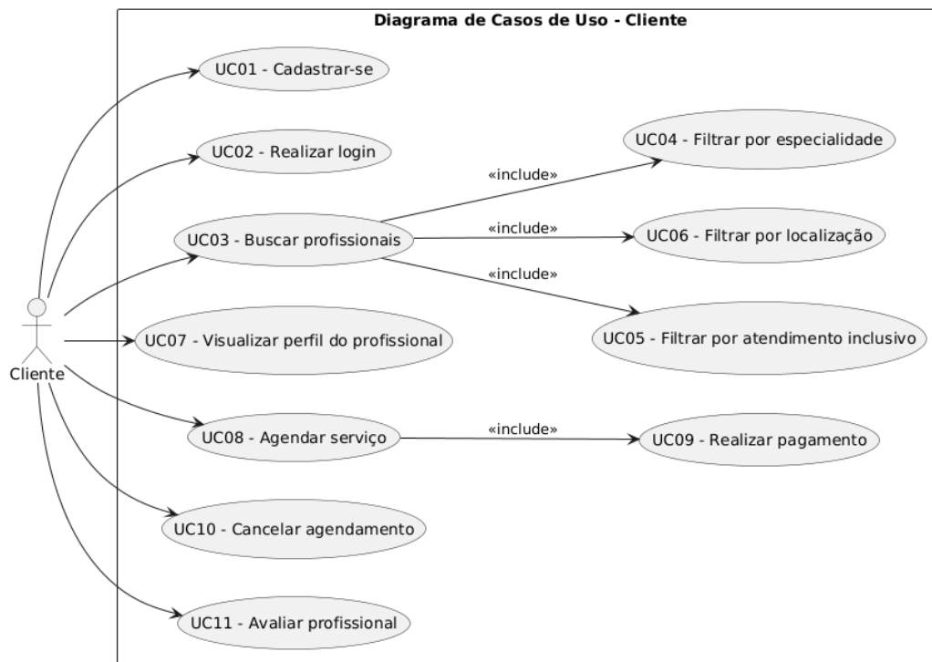
Figura 7 – Diagrama de Casos de Uso: Cliente
