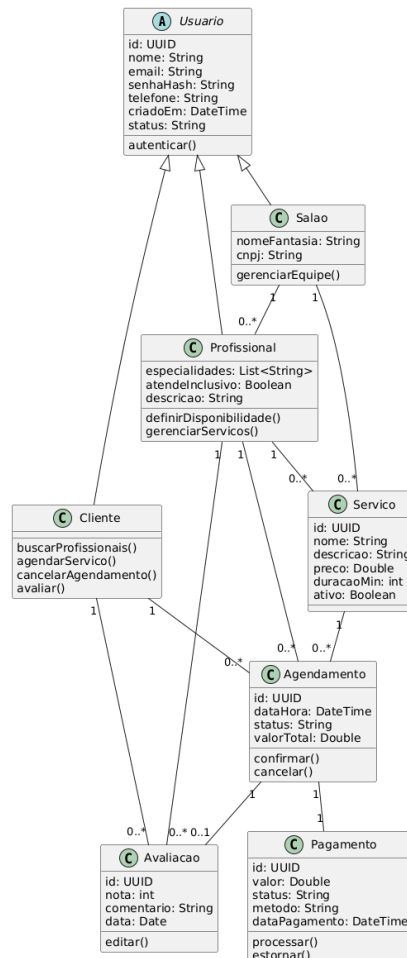
Figura 10 – Diagrama de Classes: Modelagem Leve do Sistema
