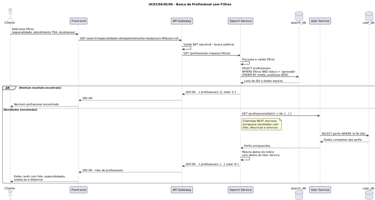
Figura 12 – diagrama de sequência: fluxo de busca de profissional
