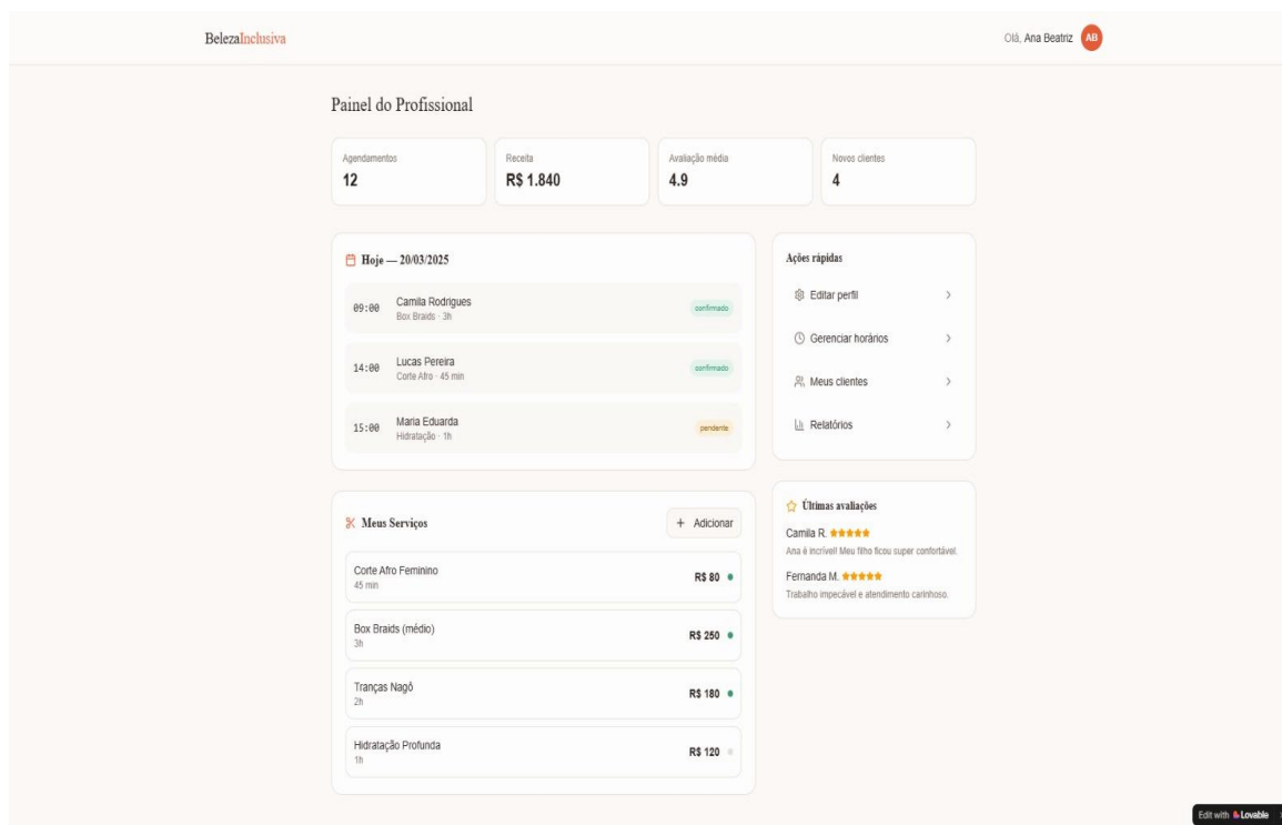
Figura 5 – Tela 5: Painel do Profissional/Salão
