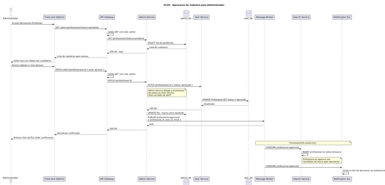
Figura 15 – diagrama de sequência: fluxo de aprovação do cadastro de profissionais por um administrador
