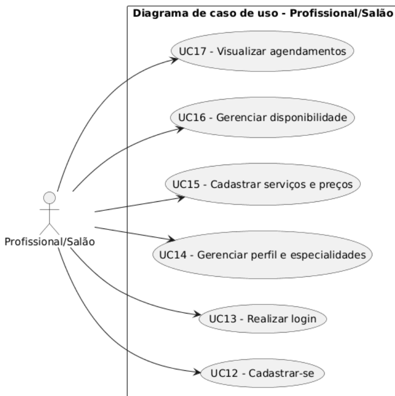
Figura 8 – Diagrama de Casos de Uso: Profissional/Salão
