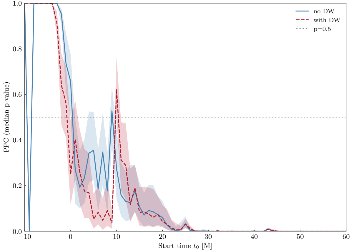
SXS:BBH:0001 — posterior predictive check
