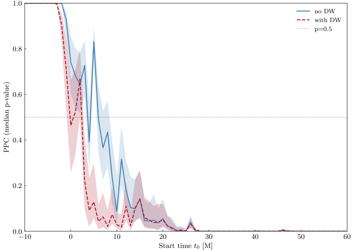
SXS:BBH:0002 — posterior predictive check
