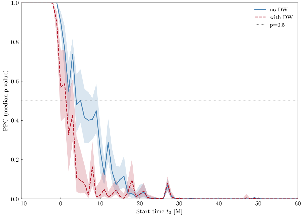
SXS:BBH:0003 — posterior predictive check
