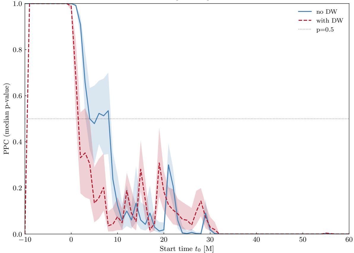
SXS:BBH:0004 — posterior predictive check
