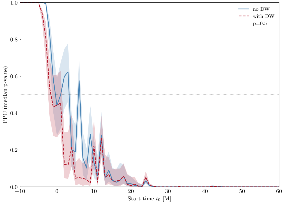
SXS:BBH:0005 — posterior predictive check
