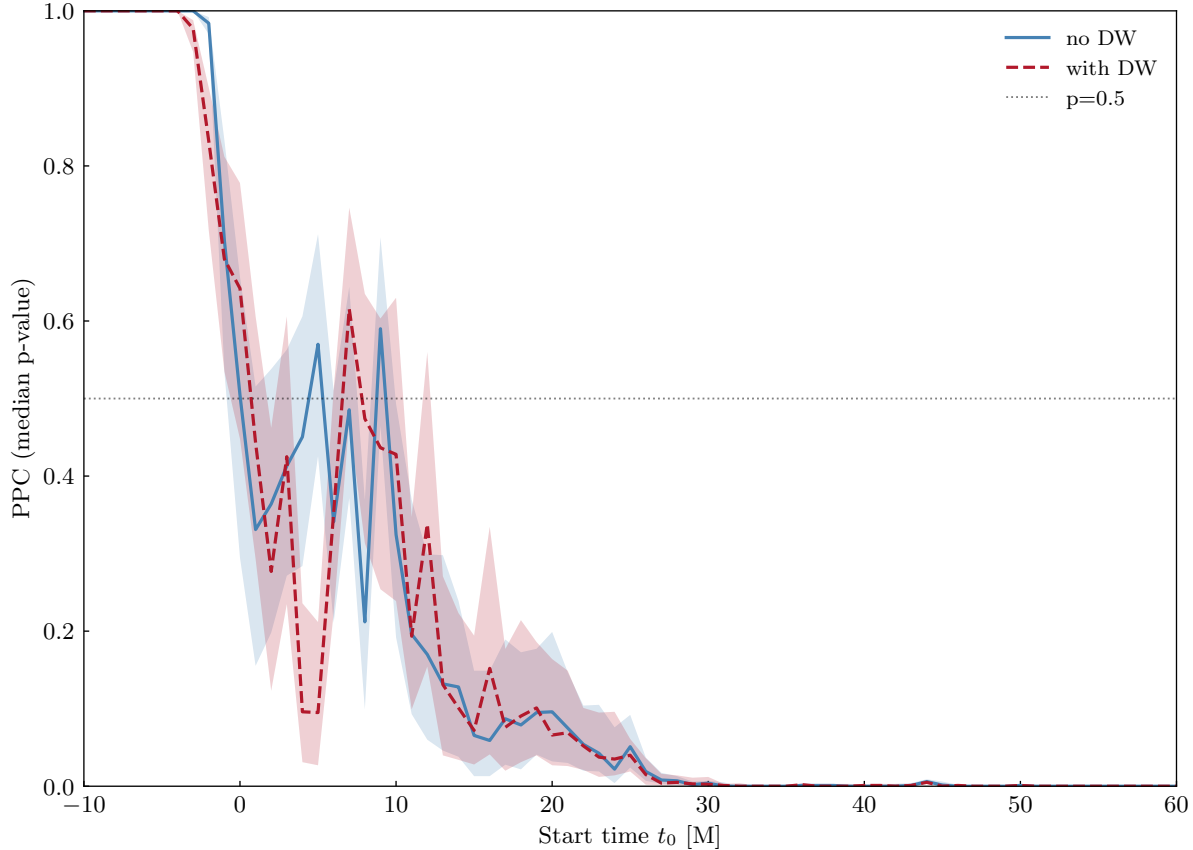
SXS:BBH:0006 — posterior predictive check
