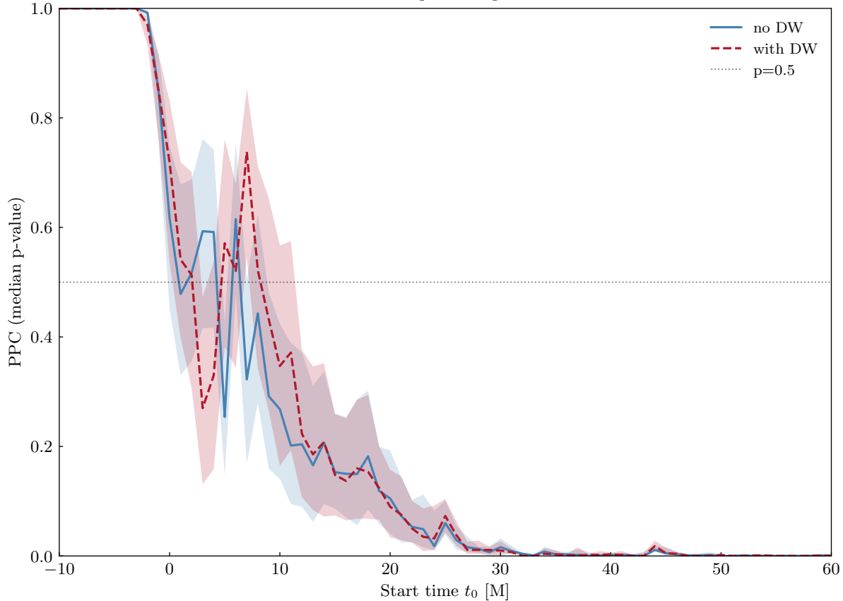
SXS:BBH:0007 — posterior predictive check
