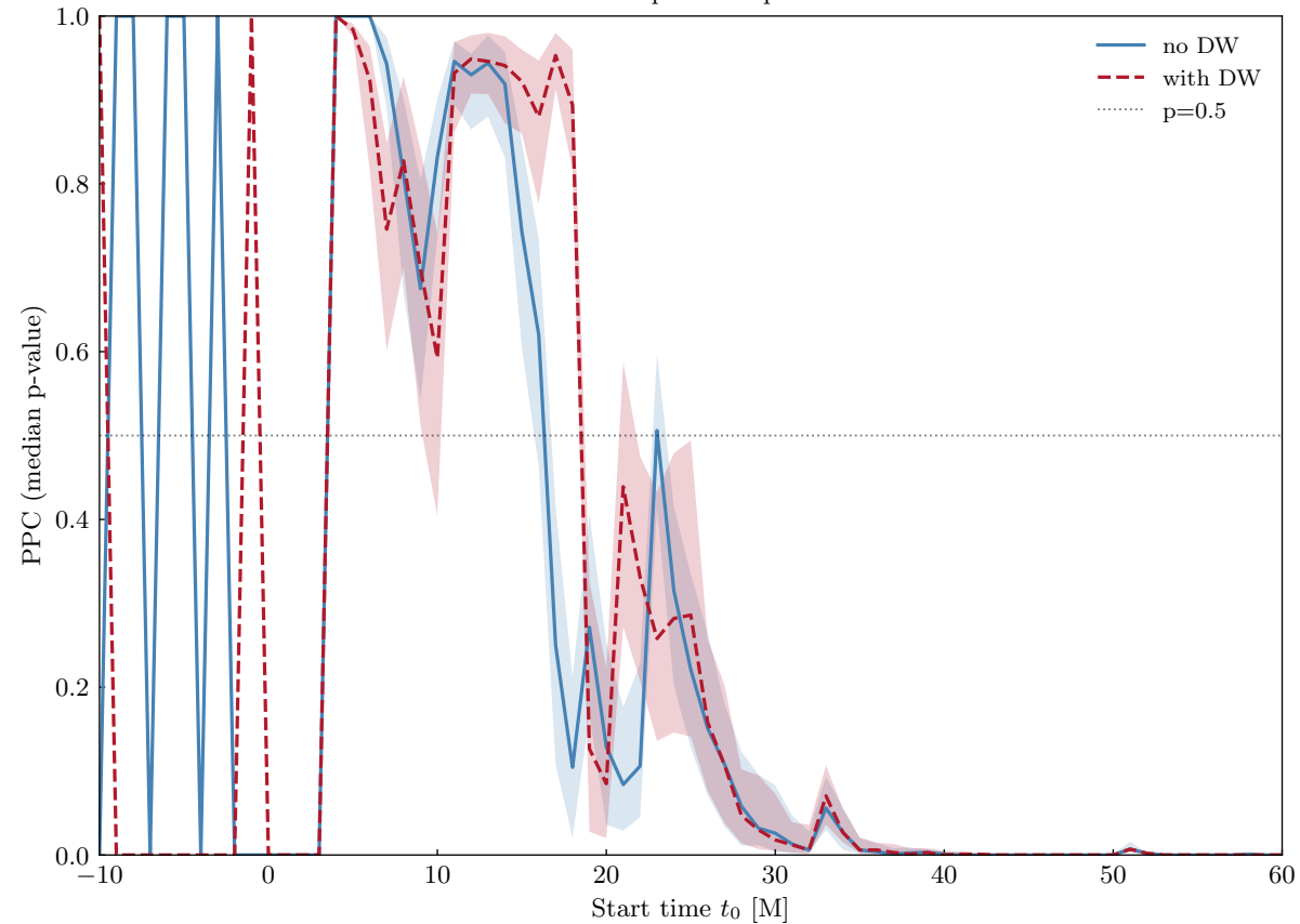
SXS:BBH:0009 — posterior predictive check
